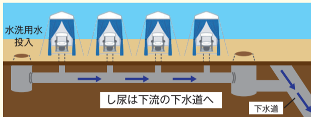
▲マンホールトイレのしくみ
