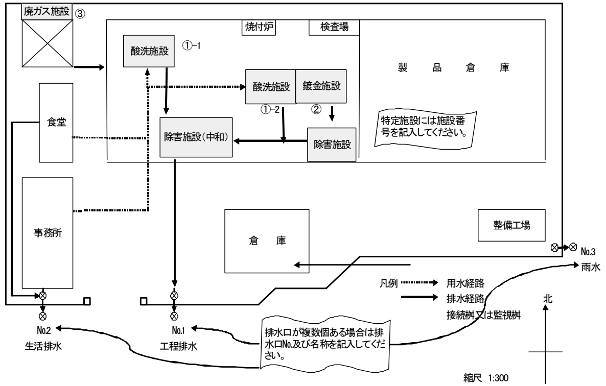
別図2 配置図
