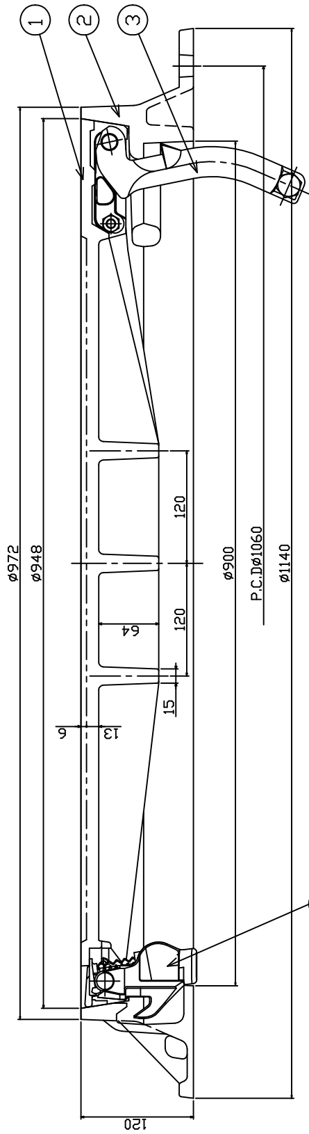
カバー、フレーム断面図
