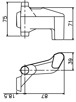
5 閉塞蓋詳細
